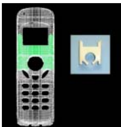
ショートショットと解析結果の比較
