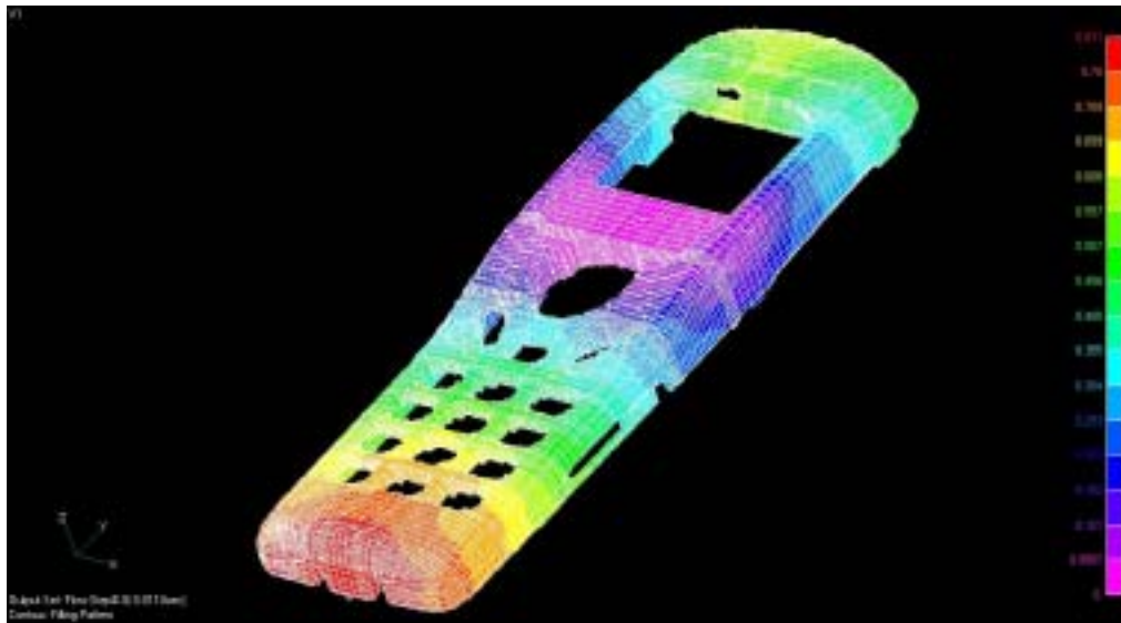
充填パターン解析結果
