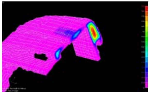
断面温度分布
